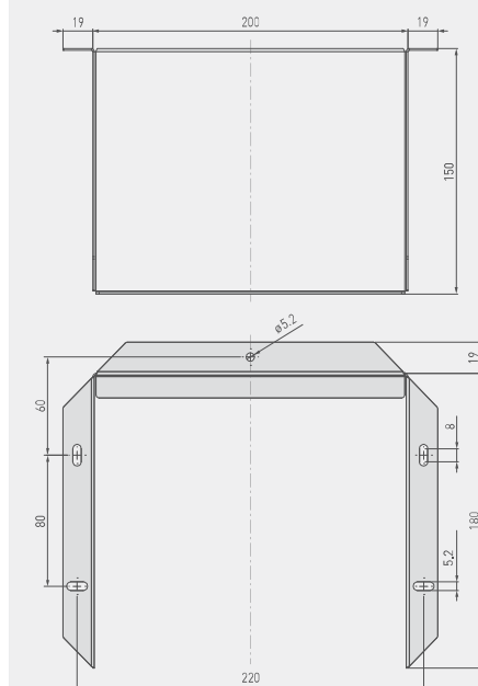
Disegno quotato
