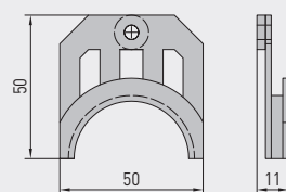
Disegno quotato
