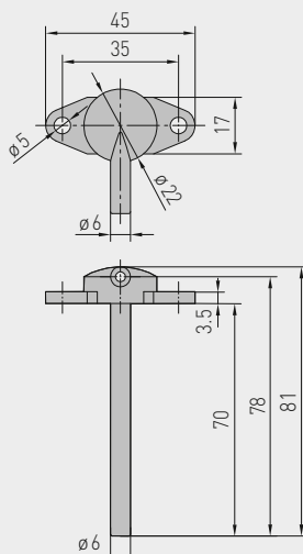
Disegno quotato
