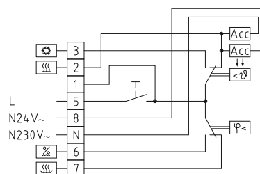
Schema di collegamento
