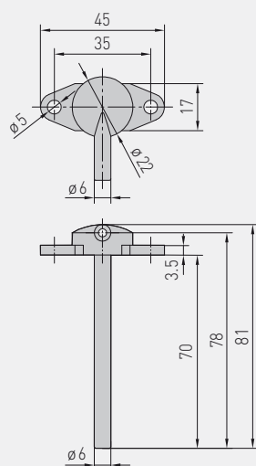
Disegno quotato ASD-07
