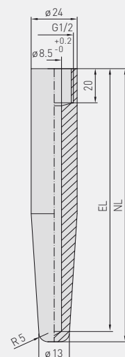
Disegno quotato ESSH
