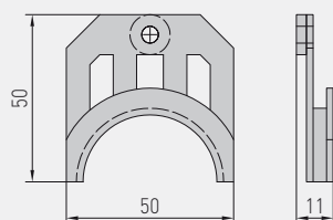
Disegno quotato MK-05-K
