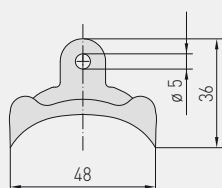
Disegno quotato MK-05-M
