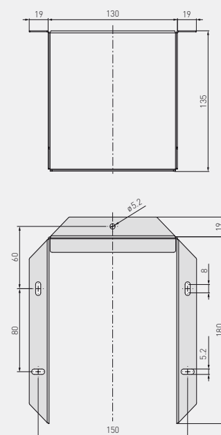
Disegno quotato
