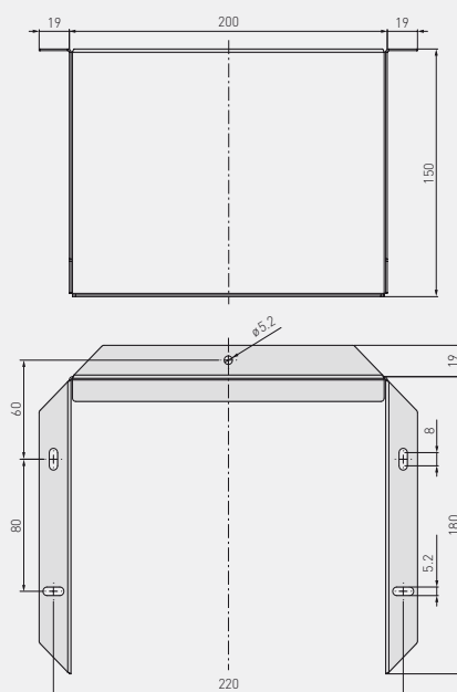
Disegno quotato
