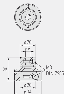
Disegno quotato TH-ADAPTER-HW
