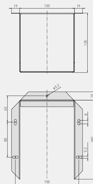
Disegno quotato
