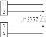
1х четырехпроводное подключение LM235Z (КР 10)
