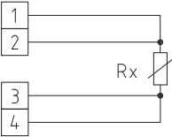
1х четырехпроводное подключение стандартное исполнение
