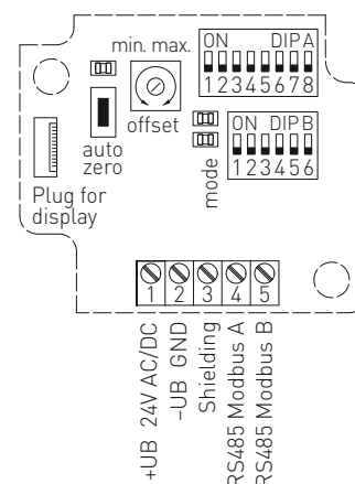
Schema di comando PREMASGARD® 121x - Modbus
