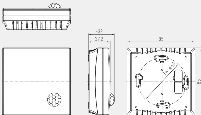
Disegno quotato
