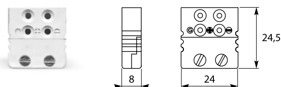
Base miniatura femmina
