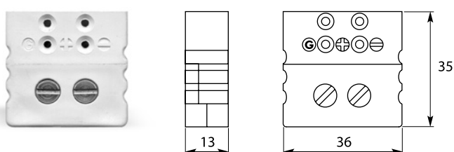
Base standard femmina
