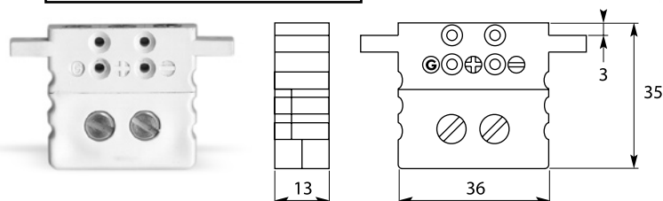
Base standard femmina
