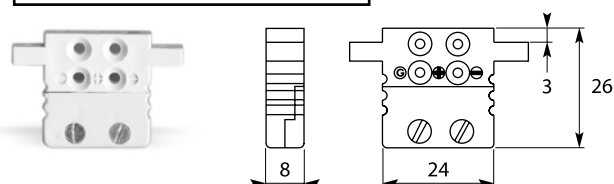
Base miniatura femmina
